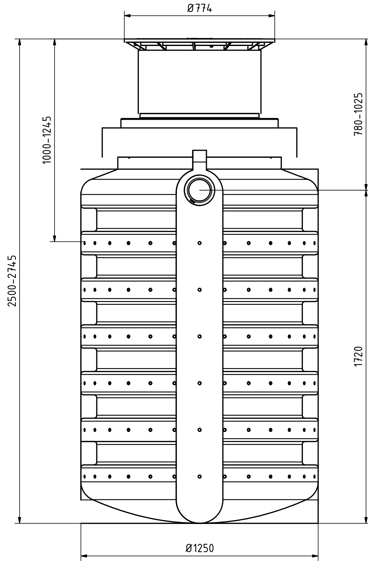
Frontansicht
